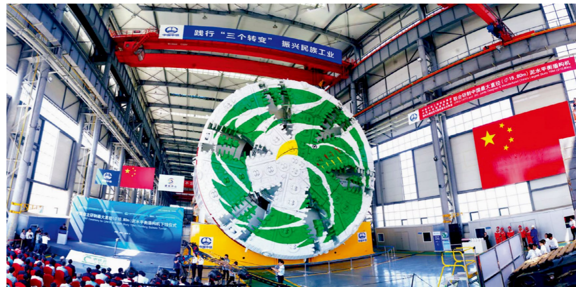
2018年9月29日，由市政总院全程参与研制的国内最大直径泥水平衡盾构机正式下线
